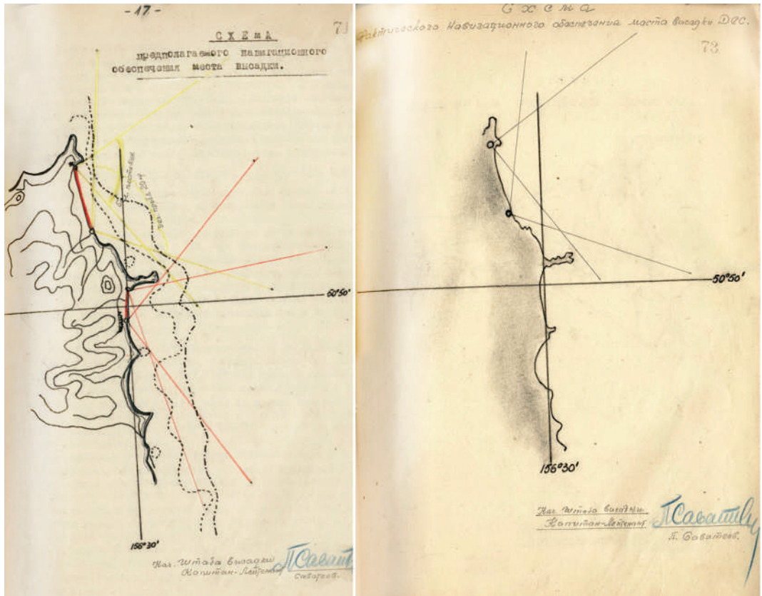
Илл. 69. Схема планируемого и фактического размещения навигационных огней на месте высадки десанта. ЦВМА
