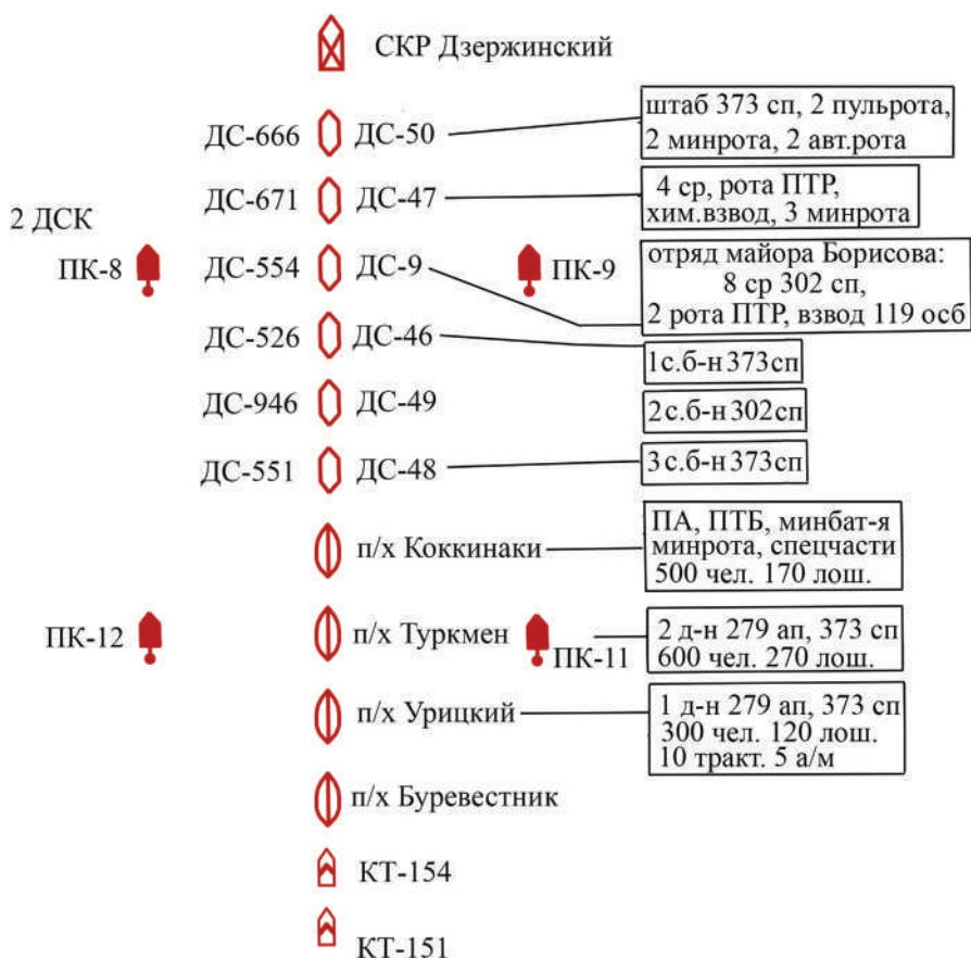
Илл. 62. Схема посадки войск второго эшелона. Рисунок автора
