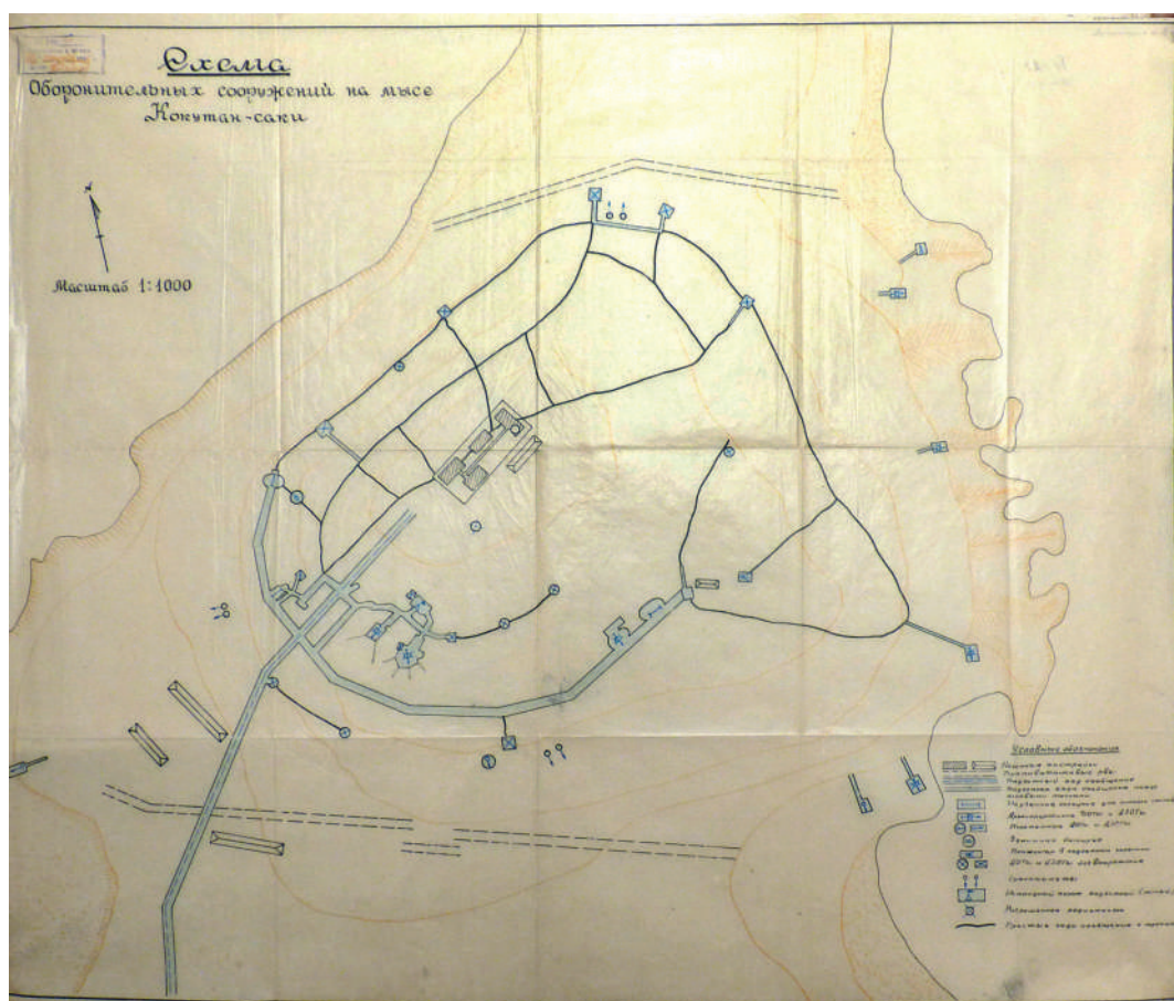
Илл. 25. План оборонительных сооружений на мысе Кокутан (мыс Курбатова). Составлен по японским данным. ЦВМА
