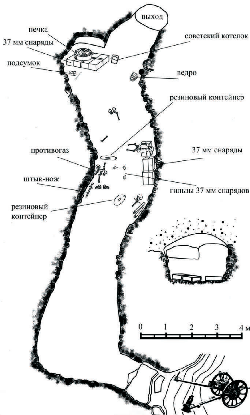
Илл. 87. Схема артиллерийской скальной огневой точки на мысе Гурьева (мыс Такэда). Рисунок автора по итогам поисковых работ 2014 года
