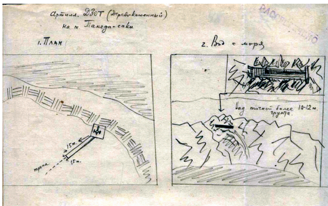
Илл. 28. Зарисовки скальной огневой точки на мысе Такэда (мыс Гурьева), выполненные сводным батальоном морской пехоты ПВМБ. ЦВМА
